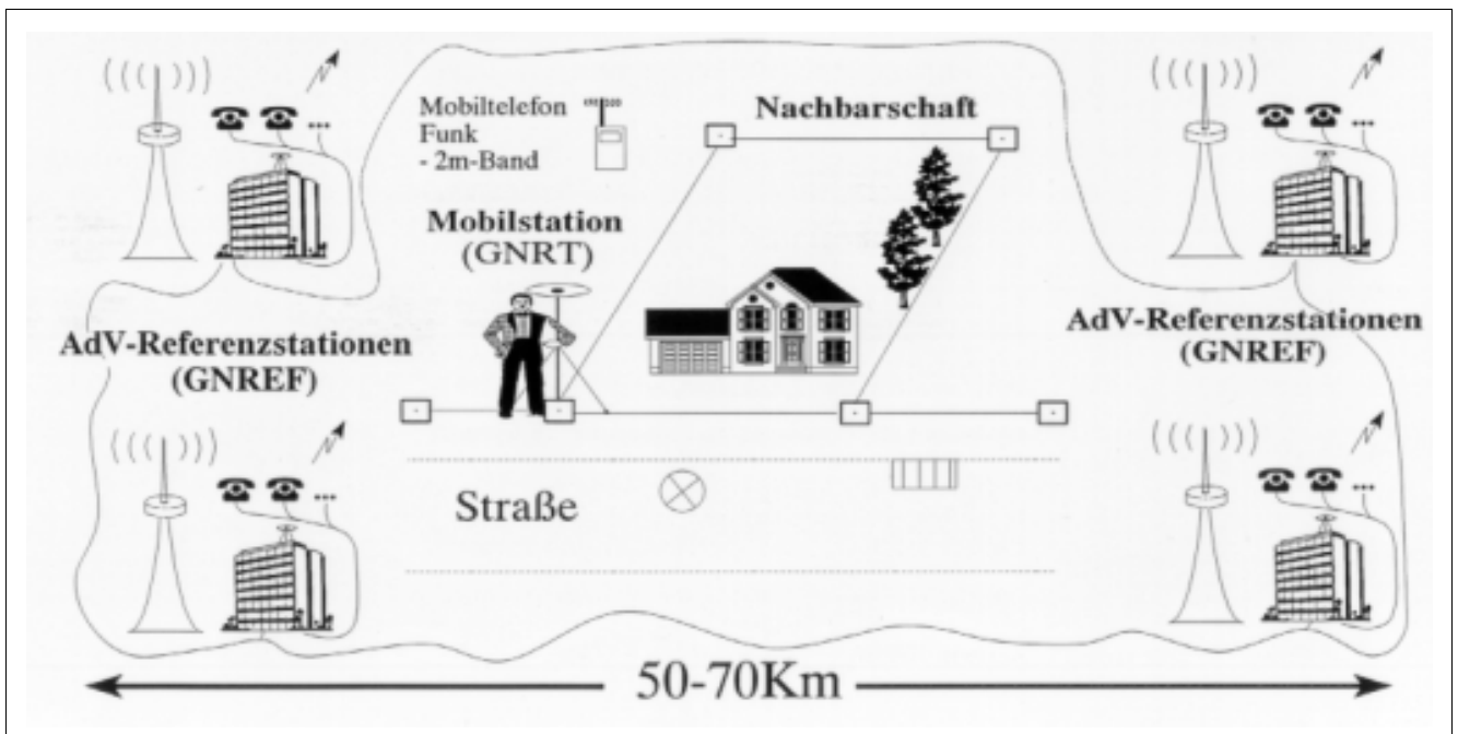
Abb. 4: GNRT im Einsatz in einem DGPS-Referenzstationsnetz
