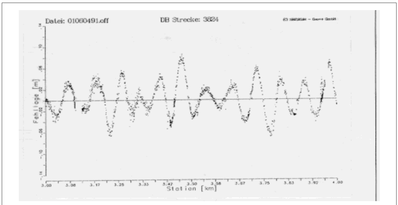
Abb. 5: Fehlloge aus einer Gleisvermessung. Die gute Übereinstimmung der beiden Kurven für Hin- und Rückweg belegt die PDGPS-Genauigkeit von wenigen Millimetern.
