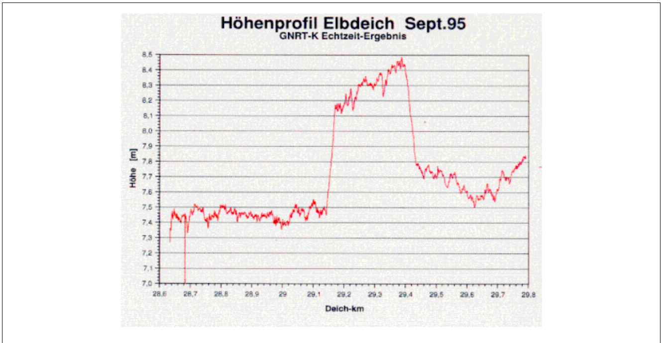
Abb. 6: Deichvermessung mit GNRT-K. Deutlich ist neben einer Erhöhung bei Deich-km 29.3 auch die Feinstruktur der Deichlinie zu erkennen.
