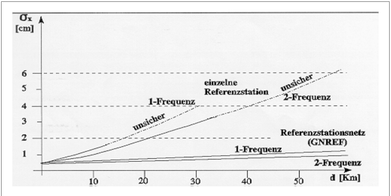
Abb. 3: Entfernungsabhängigkeit der PDGPS-Genauigkeit, unterschieden nach Empfängertyp sowie für eine einzelne Referenzstation bzw. für ein GNREF-Referenzstationsnetz.
