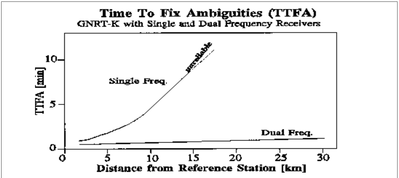
Abb. 2: Zeit bis zur Festsetzung der Mehrdeutigkeiten, für Ein- und Zweifrequenzempfänger. Zweifrequenzempfänger sind wesentlich schneller und sicherer.
