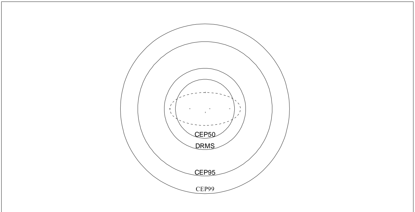
Abb. 1: Darstellung der gebräuchlichen Fehlermaße für die Lagegenauigkeit bei sonst gleichen Voraussetzungen
